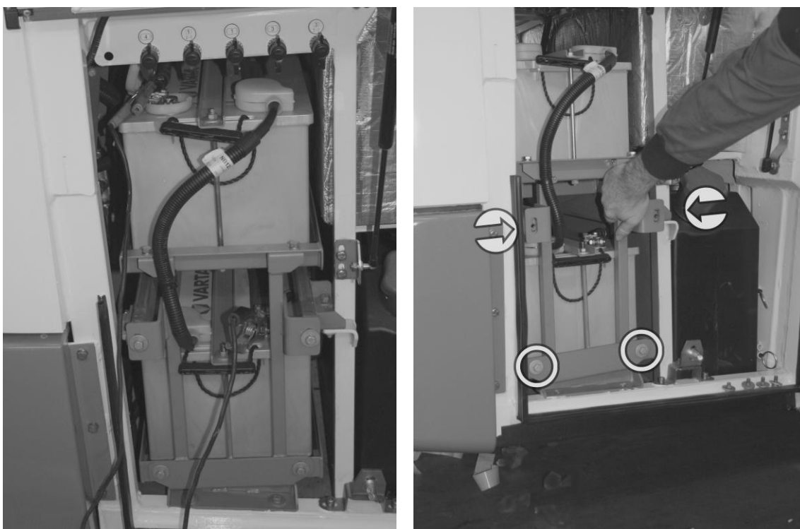
Obrázek 74: Akumulátory v poslední schráně vpravo (nízkopodlažní vůz). Pro jejich vysunutí je třeba odebrat šrouby označené šipkami. Šrouby, označené kroužkem, drží akumulátory v držáku
