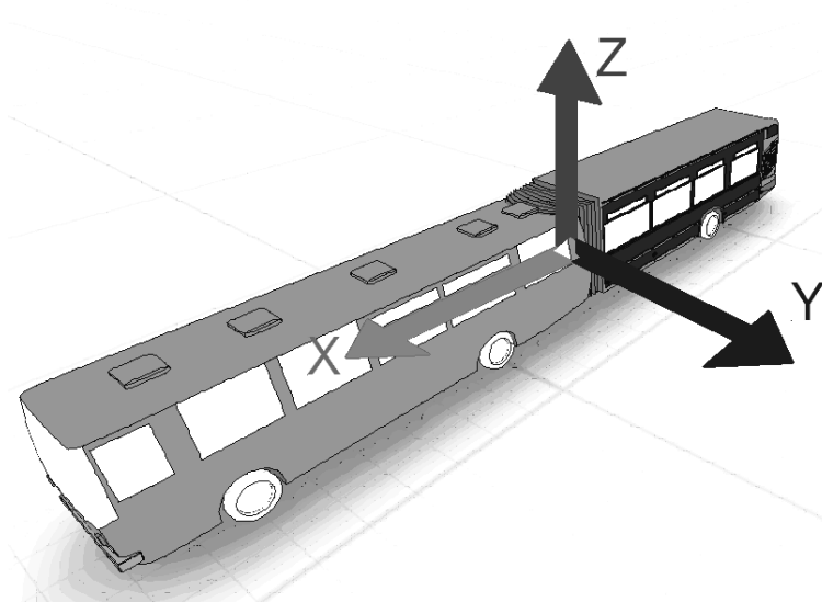
Obrázek 39: Schéma kloubového autobusu s vyznačenými směry základních os ve vztahu k spojovacímu kloubu
