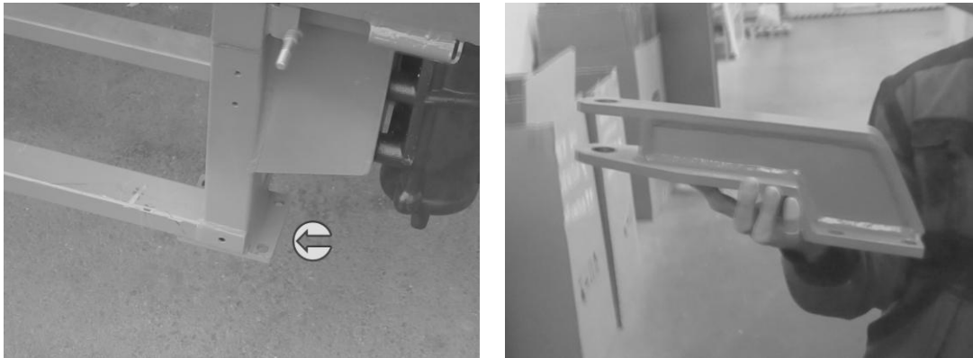
Obrázek 15: Přední vyprošťovací zařízení staršího provedení. Na snímku vlevo je přední konec roštu podvozku, kam se zařízení montuje; vpravo oko zařízení
