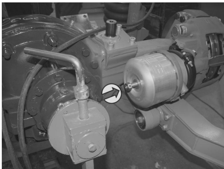
Obrázek 67: Detail brzdového válce (na nápravě před její montáží do vozu) s vytočeným šroubem nouzového odbrzdění
