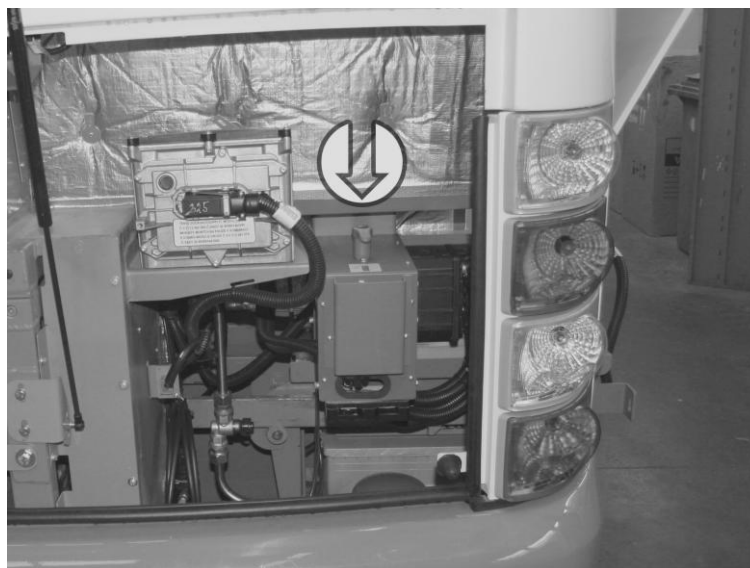
Obrázek 79: Mechanický odpojovač akumulátorů v motorovém prostoru nízkopodlažního vozu, který má akumulátory v poslední schráně na pravé straně
