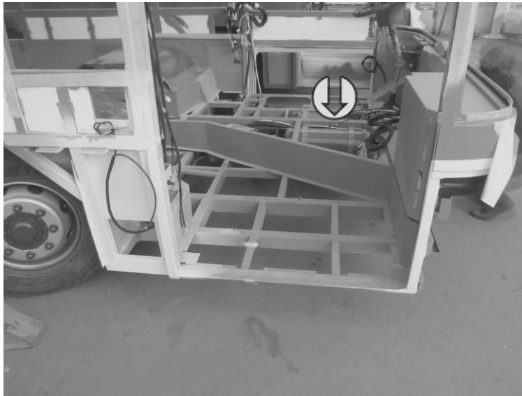
Obrázek 10: Vzduchojem uložený v roštu podvozku
