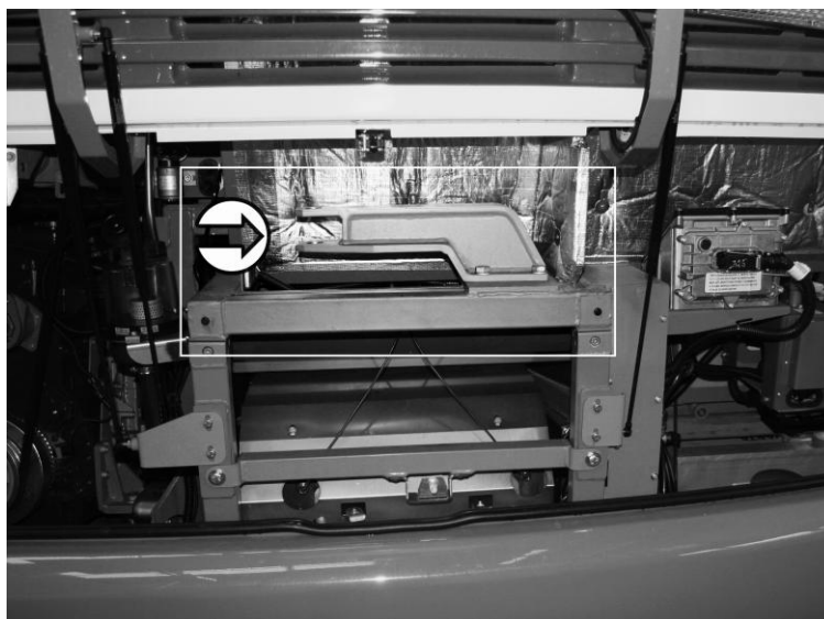
Obrázek 17: Vyprošťovací zařízení na zadní části roštu podvozku
