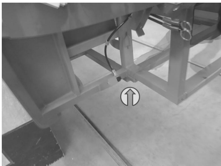
Obrázek 64: Opěrná deska pro zvedák, která má probrání pro stabilizaci horní části zvedáku. Opěra je na podélníku roštu podvozku na úrovni symbolu, který je na vnějším potahu boku vozu
