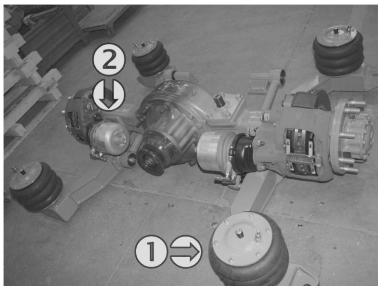
Obrázek 57: Zadní tuhá náprava před montáží do vozu. Pozicí „1“ je označen vlnovec pérování; pozicí „2“ pružinový brzdový válec (uvolňovací šroub je vytočen do odbrzděné polohy a zakryt montážní krytkou)
