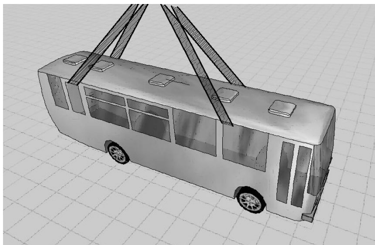
Obrázek 84: Tento způsob umístění vázacích prostředků jeřábu není vhodný
