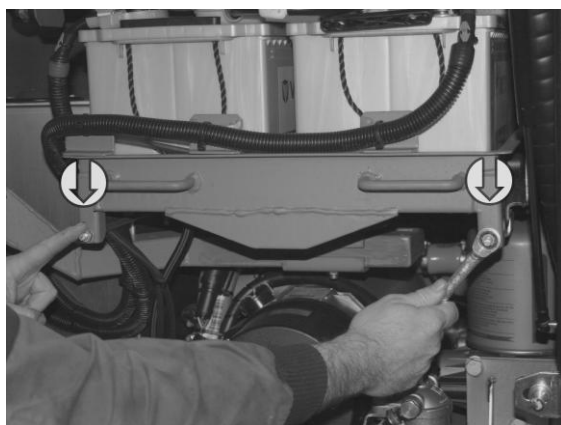
Obrázek 76: Vysouvání akumulátorů z předposlední schránky vpravo. Před vysouváním je třeba uvolnit dva zajišťovací háčky (šipky). Po vysunutí sání je možno je vytočit – obrázek vpravo
