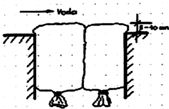
Utěšňování otvorů
